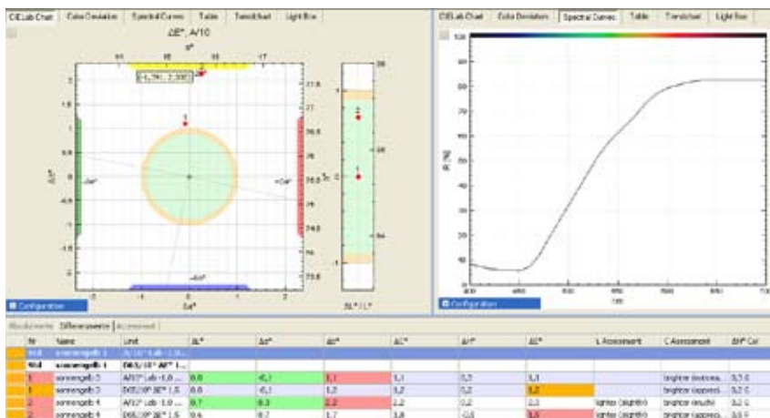
Pantalla de Control de Calidad con tabla de valores incluyendo la visualización de pasa no-pasa, tolerancia y con 6 opciones de pantalla elegibles.
